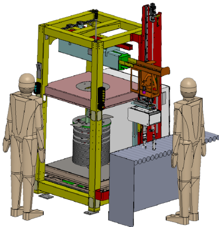
Kalibreringstester
